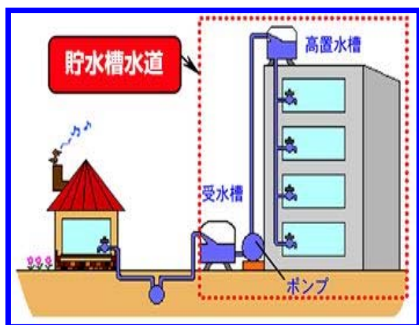
図-3.6.2 貯水槽水道の概念図
