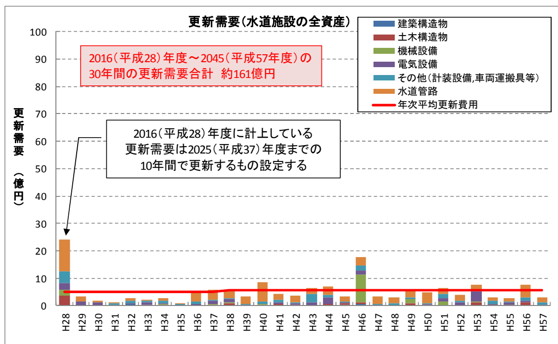
図-4.5.2 シミュレーションにおける更新需要見通し (大牟田市が目標とする更新基準を迎えた時点で更新した場合)
