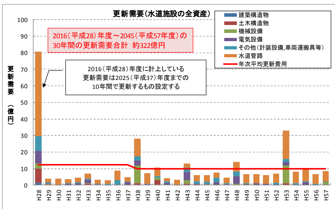
図-4.5.1 シミュレーションにおける更新需要見通し （法定耐用年数を迎えた時点で更新した場合）
