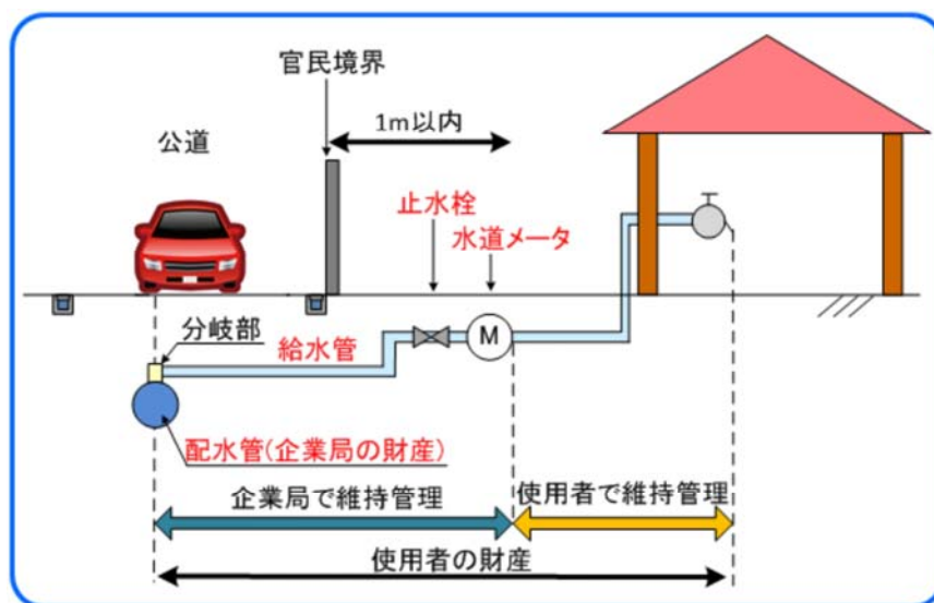
図-3.6.1 給水装置における維持管理範囲の概念図
