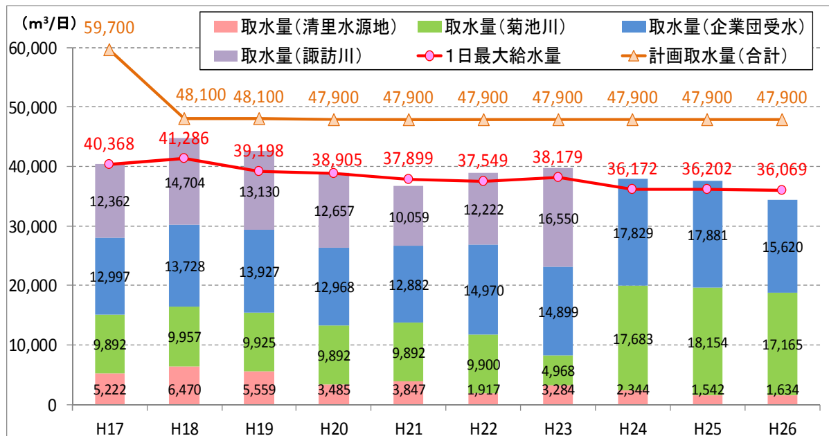
図-3.3.2 水源別取水量・計画取水量・1日最大給水量
