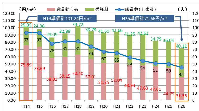
図-3.9.2 有収水量1m³当たりの人件費及び委託料の推移
