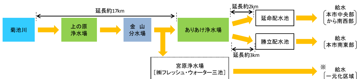
図-3.4.2 取水～送水概念図
