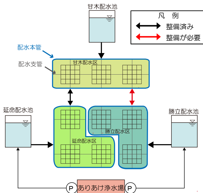
図-4.3.2 配水区域間の相互融通概念図（将来計画）
