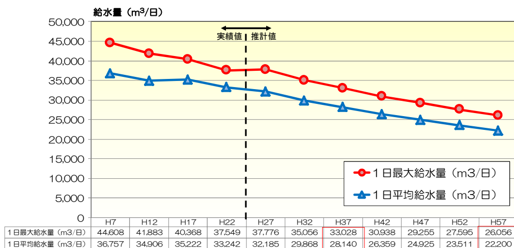
図-4.1.2 給水量の予測
