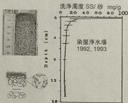
図30 上田市のろ過池での砂層断面
