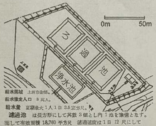
図8 創設当時の染屋浄水場
