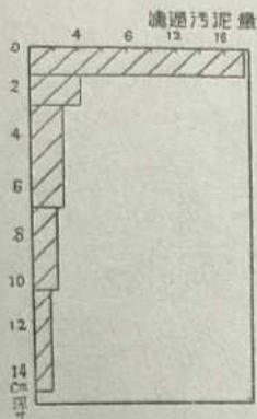
図22 東京のろ過池砂層の状態（昭和17年）
