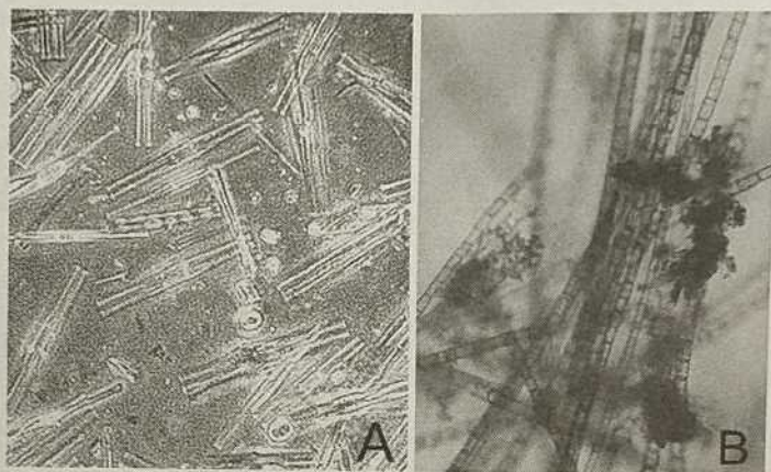
図29 境浄水場の針珪藻 (A) と染屋浄水場の糸状珪藻 (B)
